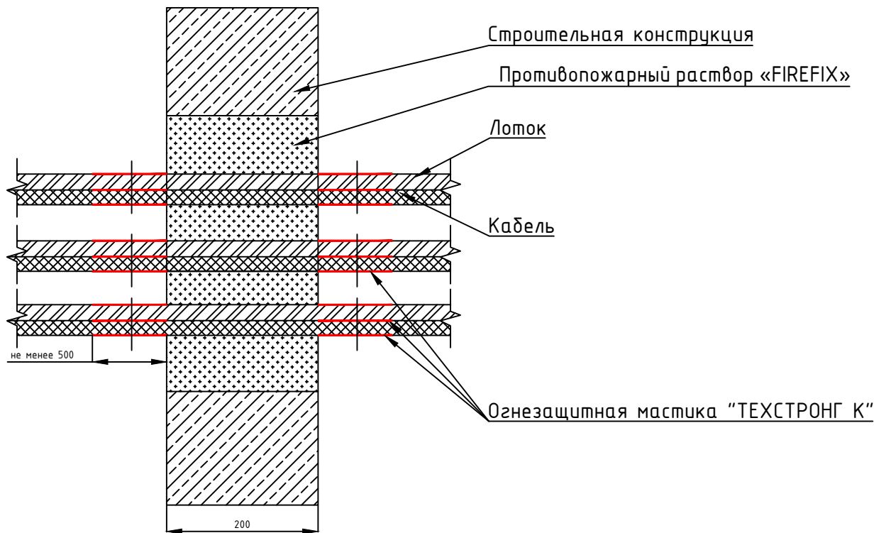
Разрез 1-1
