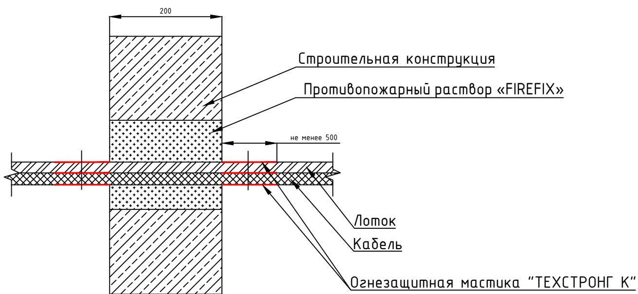
Разрез 1-1
