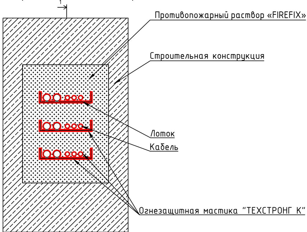
Разрез 1-1
