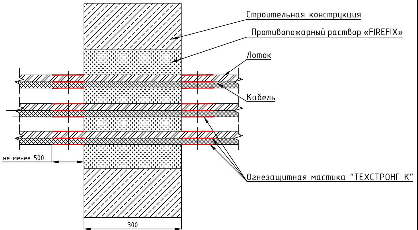
Разрез 1-1
