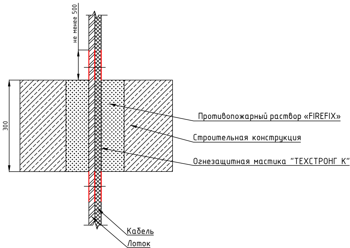
Разрез 1-1
